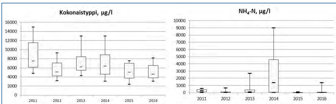
Kuva 4.11. Kokonaistypen ja ammoniumtyypen pitoisuudet Arolamminkoskessa (V84) vuosina 2011-2016. Kuvan laatikkokaaviossa laatikon alareuna vastaa alaneljännestä, yläreuna yläneljännestä, alin ja ylin poikkiviiva ovat aineiston pienin ja suurin arvo ja laatikossa oleva poikkiviiva on mediaani. Havaintoja oli vuosittain vähintään 12.
