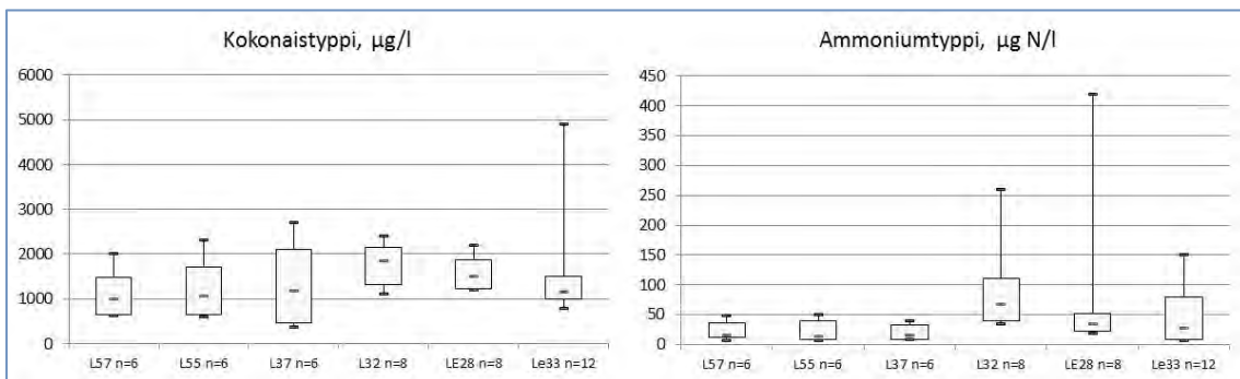
Kuva 4.40. Tyyppipitoisuudet Klaukkalan puhdistamon vaikutusalueella (L32 ja Le28) sekä vertailualueilla (L37 ja Le33) vuonna 2016. Kuvan laatikkokaaviossa laatikon alareuna vastaa alaneljännestä, yläreuna yläneljännestä, alin ja ylin poikkiviiva ovat aineiston pienin ja suurin arvo ja laatikossa oleva poikkiviiva on mediaani.
